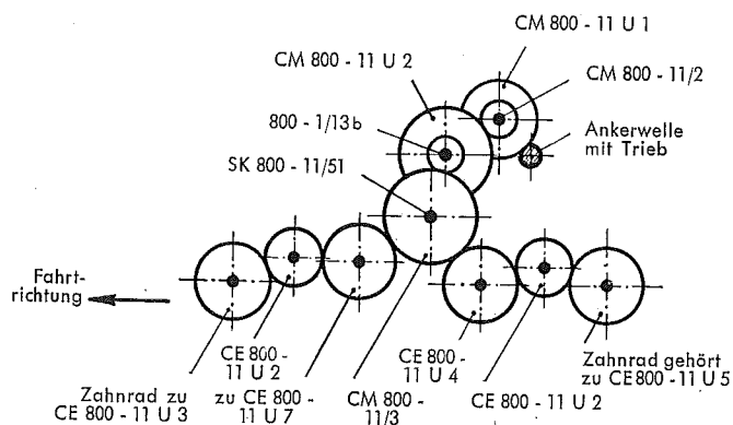
Fig. 4 Anordnung der Getrieberäder
