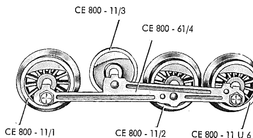
Fig. 6 Treibräder auf der Bürstenseite, bestehend aus:
