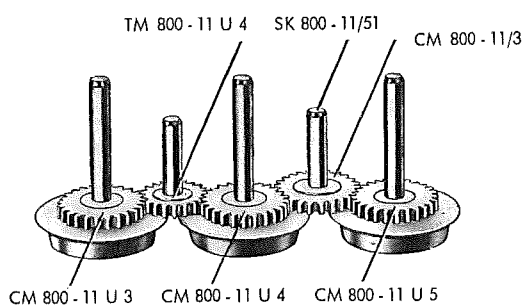
Fig. 5 Treibachsenteile auf der Getriebeseite
