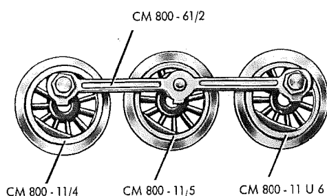
Fig. 7 Gestänge bestehend aus:
