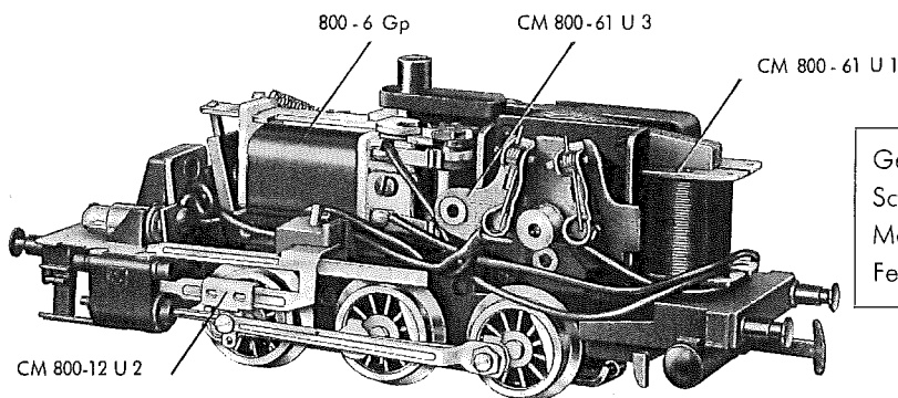
Fig. 2 Fahrgestell (Bürstenseite)
