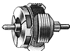
Fig. 10 Anker 3polig mit Kollektor
