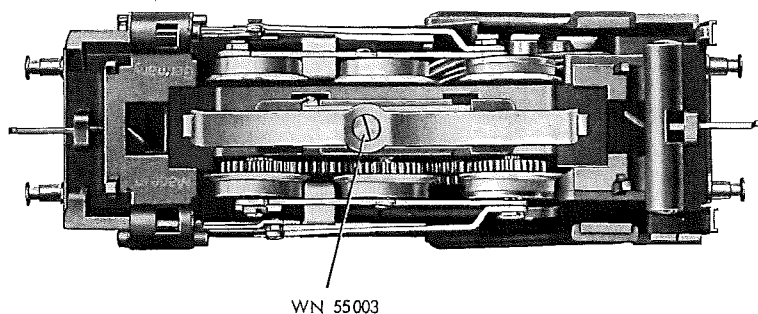
Fig. 2b Fahrgestell von unten gesehen
