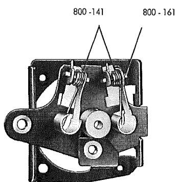
Fig. 11 Motorschild
