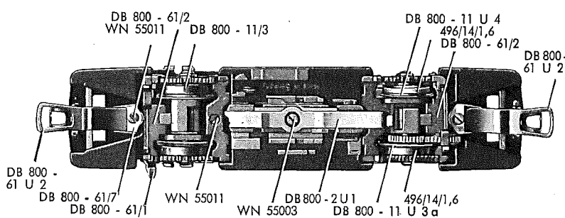
Fig. 4 Anordnung des Antriebes
