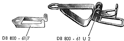
Fig. 8 Achslager
