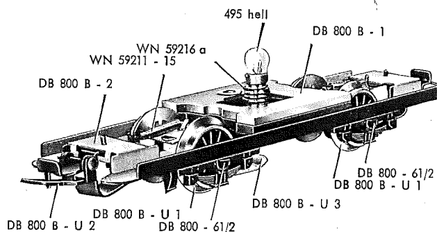
Fig. 10 Fahrgestell für Beiwagen-Aufbau
