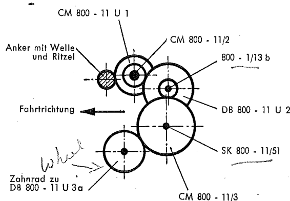
Fig. 4 Anordnung des Antriebes
