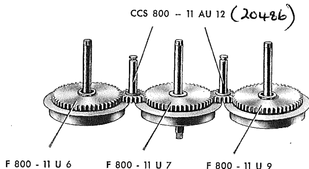
Fig. 7 RADSATZ auf der Bürstenseite bestehend aus:
