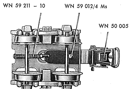
Fig. 4 DREHGESTELL mit Kupplung
