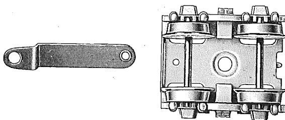
Fig. 4 DREHGESTELL mit Kupplung
