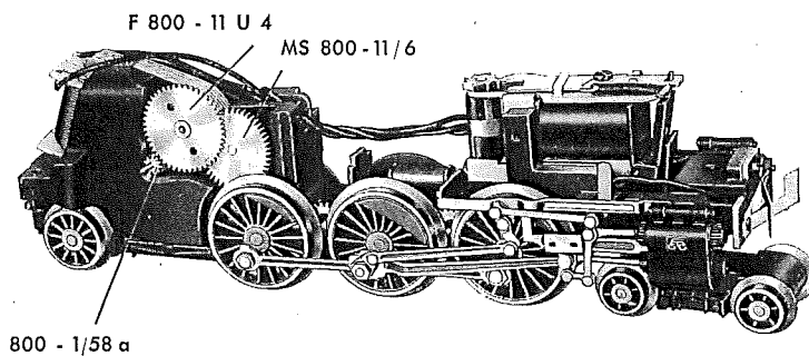
Fig. 2a FAHRGESTELL von vorne gesehen
