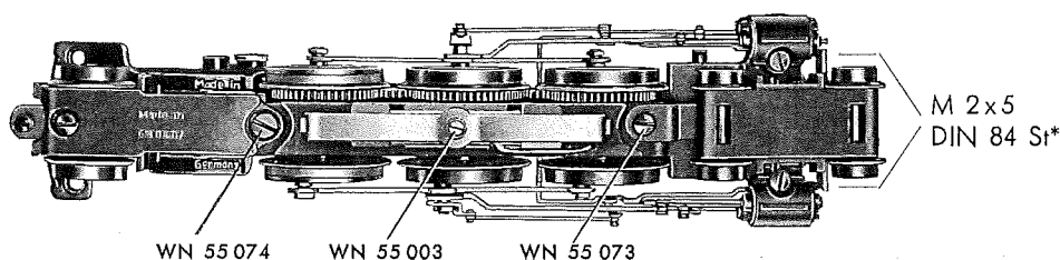
Fig. 2 b FAHRGESTELL von unten gesehen
