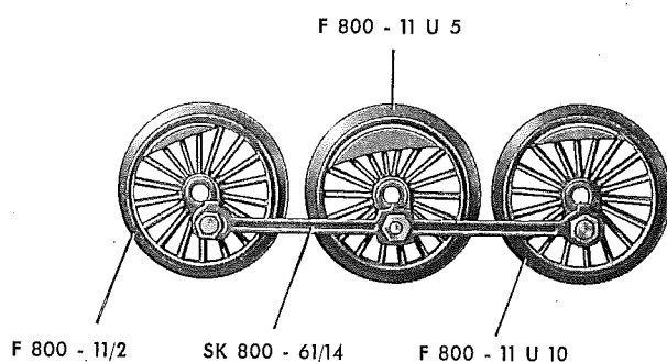
Fig. 8 GESTÄNGE (Heusinger-Steuerung) bestehend aus:
