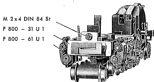
Fig. 2a FAHRGESTELL von vorne gesehen
