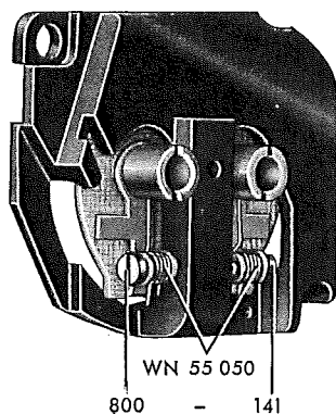
Fig. 15 MOTORSCHILD
