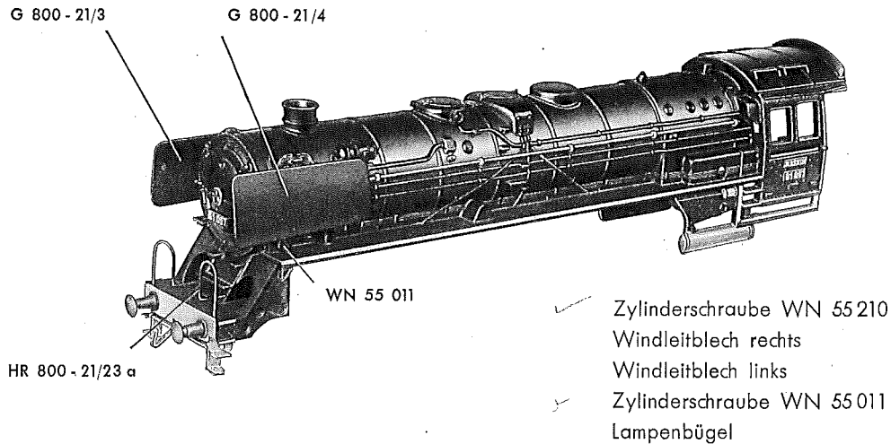
Fig. 1 LOKOMOTIV-AUFBAU
