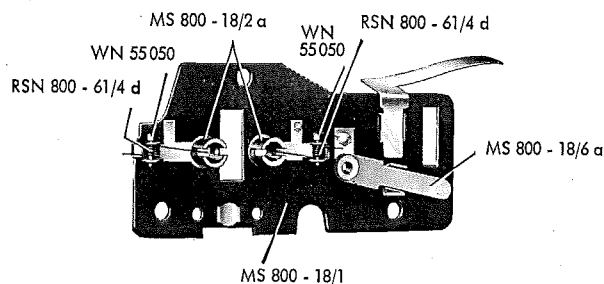
Fig. 4 Schalttafel
