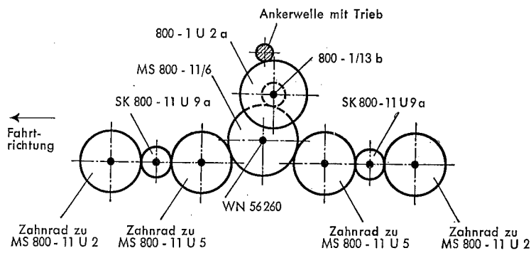
Fig. 6 a Treibradsatz
