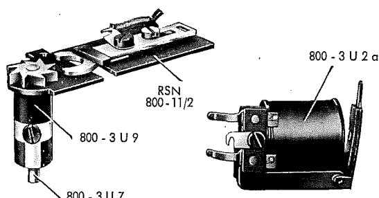
Fig. 10 Schaltautomat
