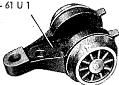
Fig. 8 Laufgestell
