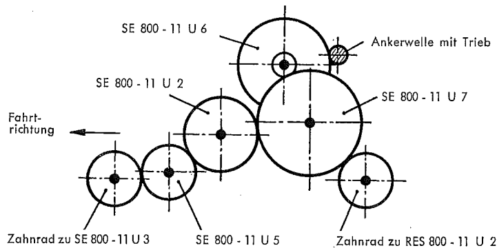
Fig. 8 Treibachsenteile auf der Getriebeseite
