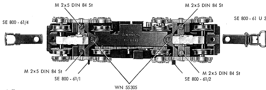
Fig. 3 Traggestell
