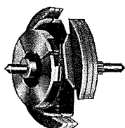
Fig. 12 Anker dreipolig mit Kollektor
