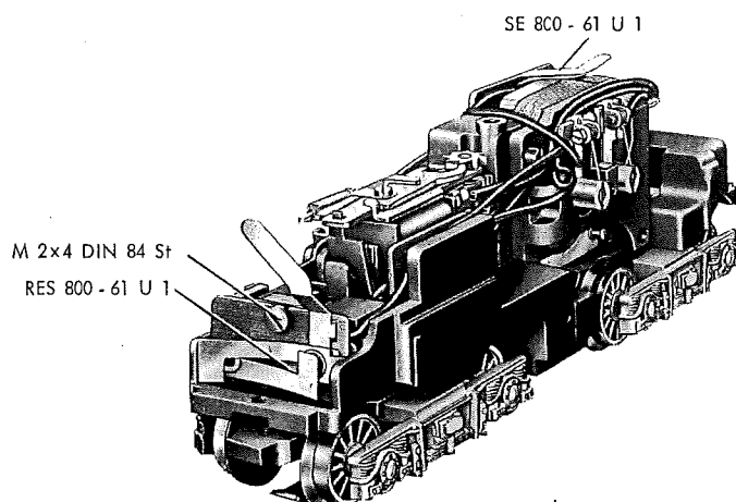
Fig. 2a Fahrgestell von vorne gesehen
