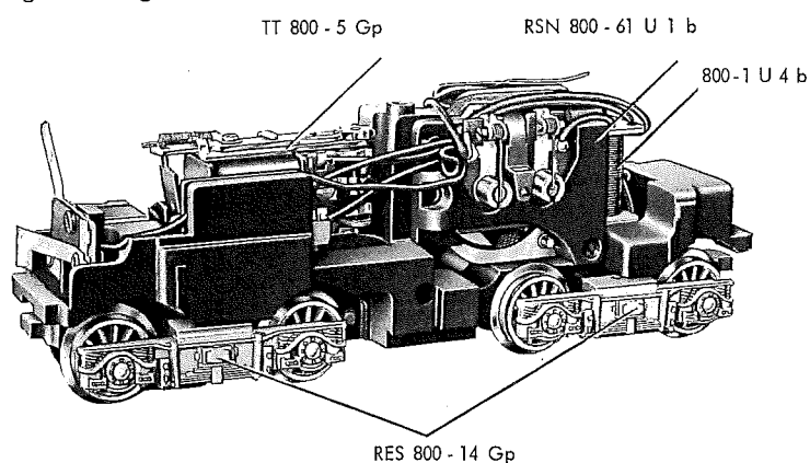
Fig. 2a Fahrgestell von vorne gesehen
