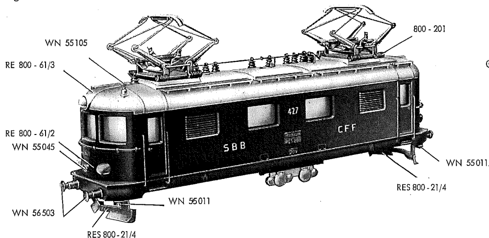
Fig. 1a Scherenstromabnehmer
