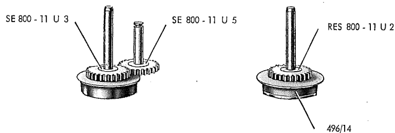
Fig. 9 Treibräder auf der Bürstenseife
