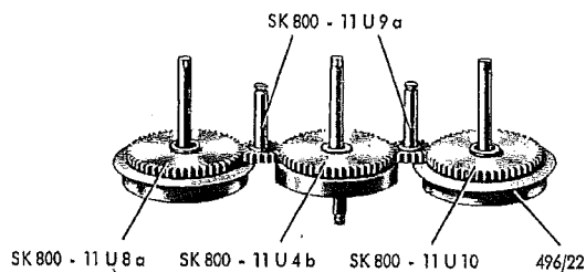
Fig. 7 Treibachsenteile auf der Getriebeseite bei SK 800 N und HR 800 N
