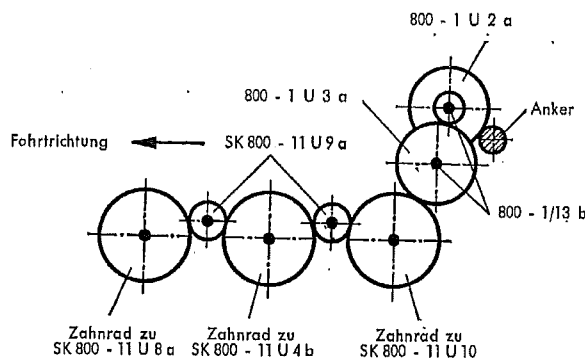
Fig. 6 Anordnung der Getrieberäder bei SK 800 N und HR 800 N
