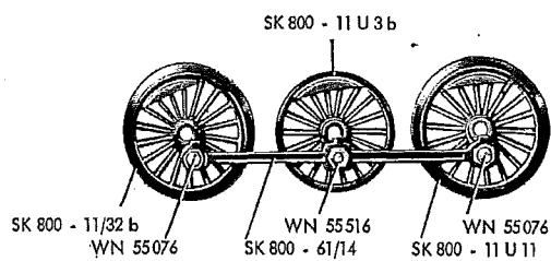
Fig. 8 Treibräder auf der Bürstenseite bei SK 800 N und HR 800 N
