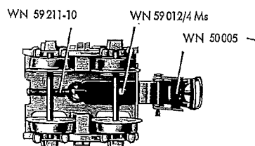
Fig. 4 Drehgestell (mit Kupplung) für SK 809 N und HR 809 N
