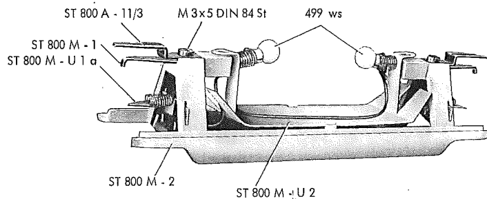
Fig. 8a Übertrager
