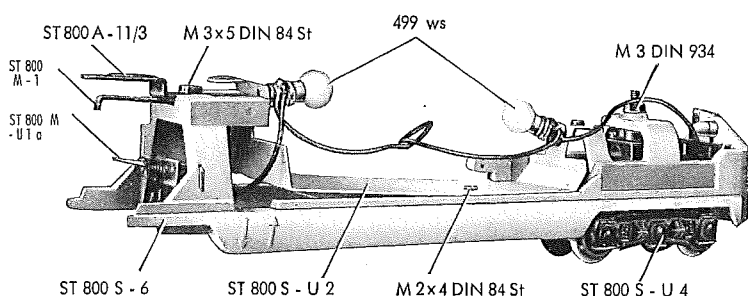
Fig. 11 Hinteres Fahrgestell
