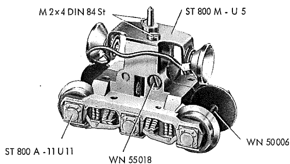
Fig. 9 Drehgestell mit Doppellichtkupplung
