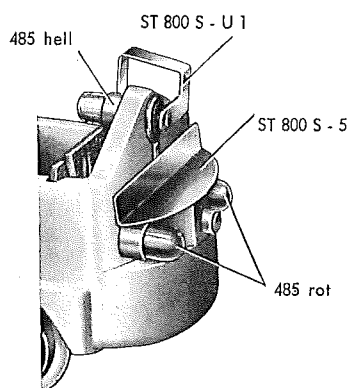
Fig. 11a Endbeleuchtung
