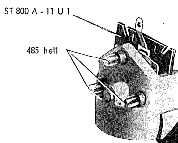
Fig. 3 Vordere Federplatte
