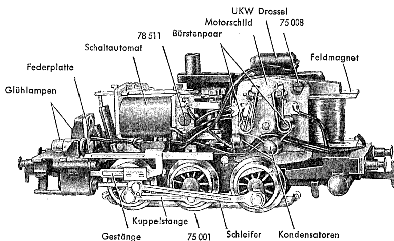
Fig. 2 Fahrgestell
