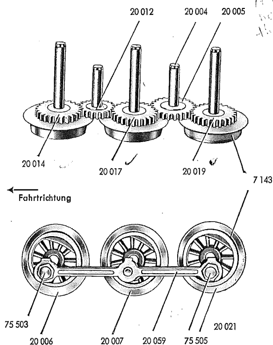
Fig. 6 Gestänge
