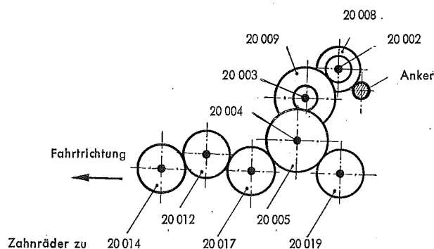
Fig. 5 Treibachsenteile und Treibräder
