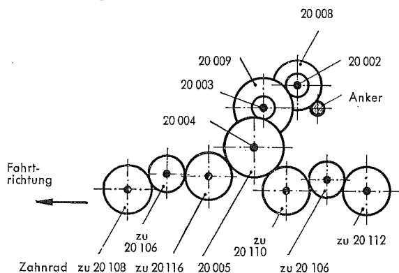
Fig. 4 Anordnung der Getrieberäder
