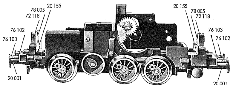
Fig. 4 Anordnung der Getrieberäder
