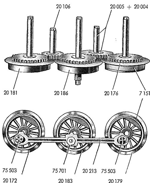
Fig. 5 Treibachsenteile und Treibräder
