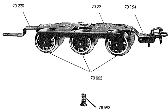
Fig. 2 Fahrgestell
