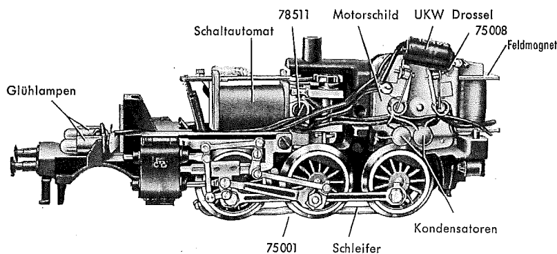
Fig. 2 Fahrgestell
