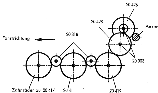
Fig. 4 Anordnung der Getrieberäder
