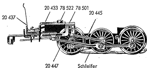
Fig. 2b Bodenstück mit Gestänge
