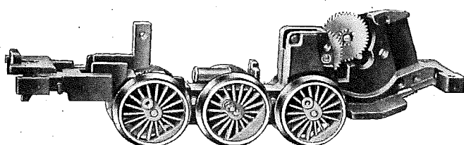
Fig. 3 Treibgestell
