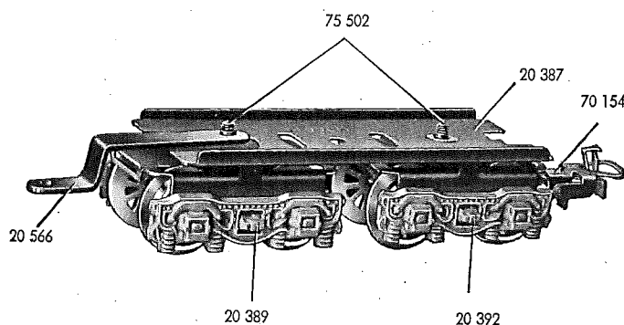
Fig. 2 Fahrgestell
