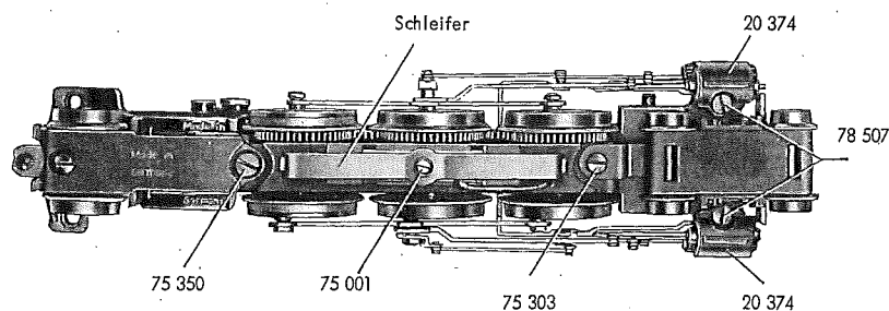
Fig. 3 Treibgestell
