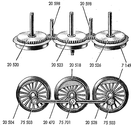
Fig. 6 Gestänge
