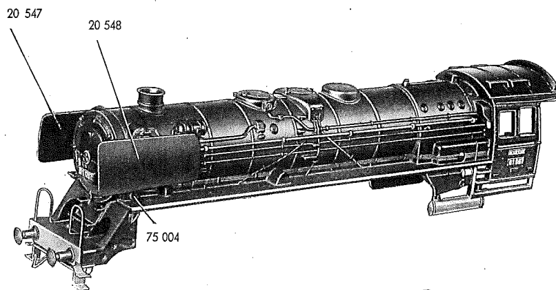
Fig. 1 Lokomotiv-Aufbau
