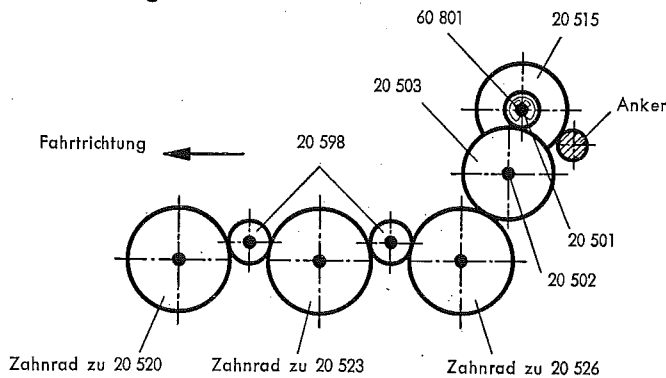
Fig. 5 Treibachsenteile und Treibräder
