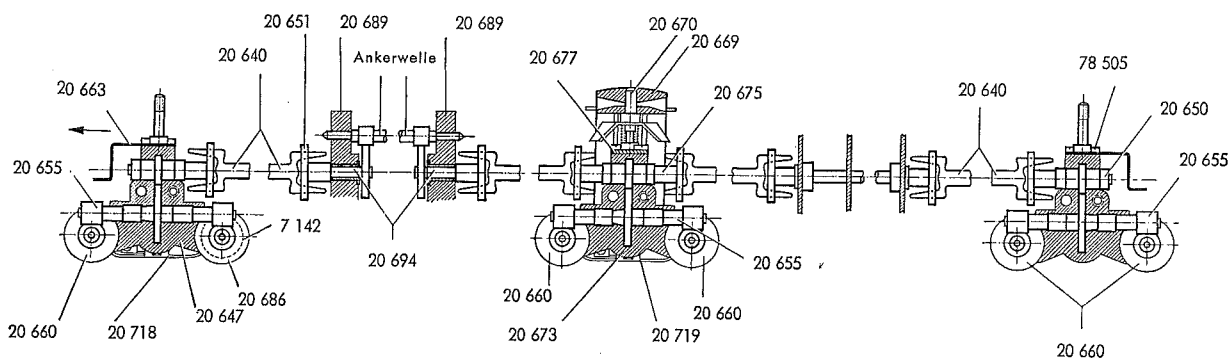
Enddrehgestell ohne Schleifer 20 722
