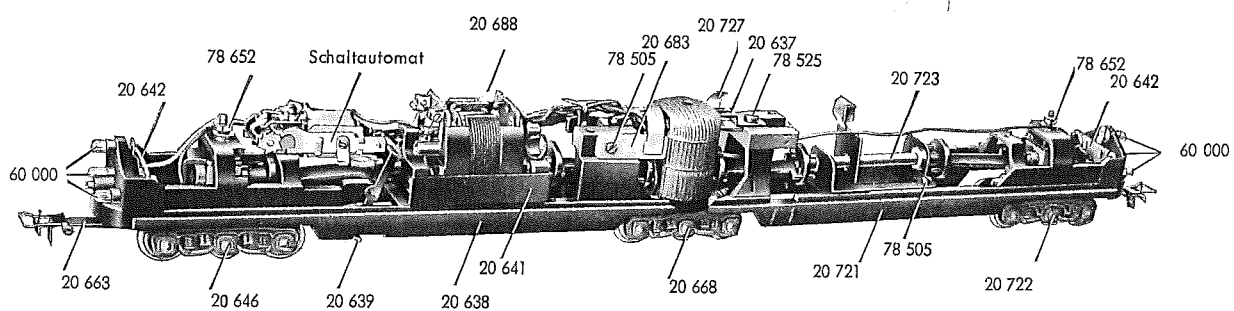
Hinteres Fahrgestell 20 720
