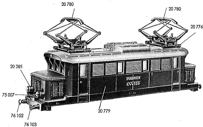
Fig. 1 Lokomotiv-Aufbau
