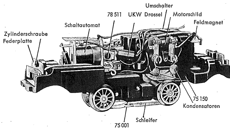
Fig. 2 Fahrgestell
