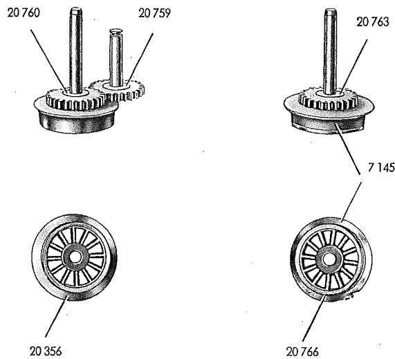
Fig. 6 Laufgestell
