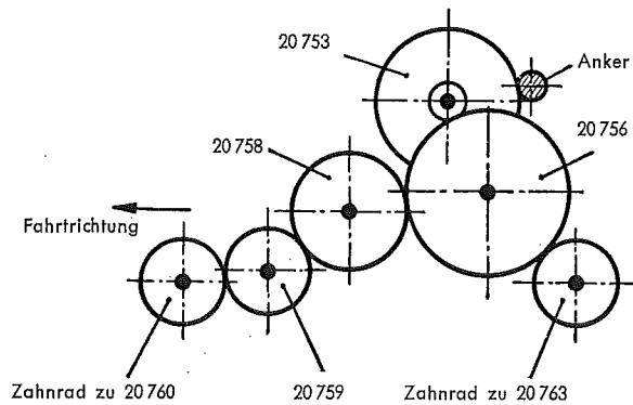
Fig. 5 Treibachsenteile und Treibräder
