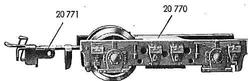
Fig. 6 Laufgestell
