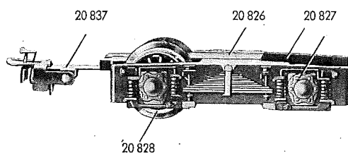
Fig. 6 Laufgestell
