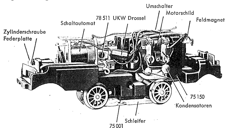
Fig. 2 Fahrgestell
