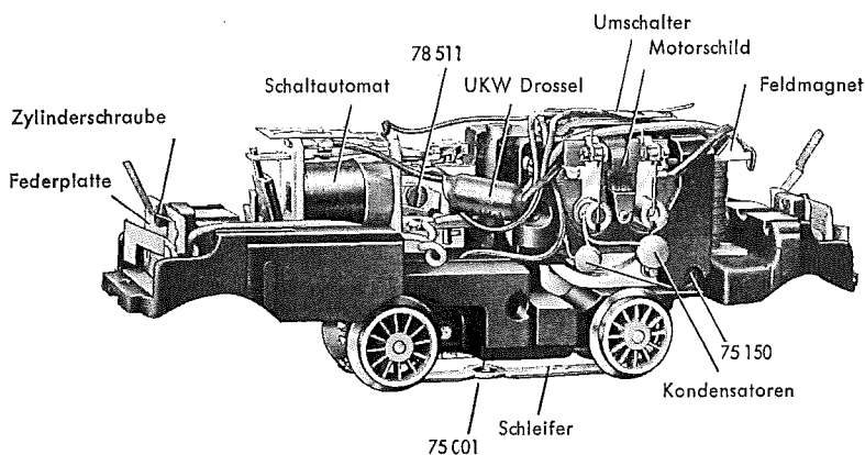
Fig. 3 Treibgestell
