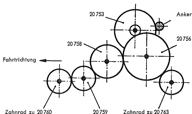
Fig. 5 Treibachsenteile und Treibräder
