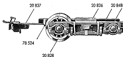
Fig. 6 Laufgestell
