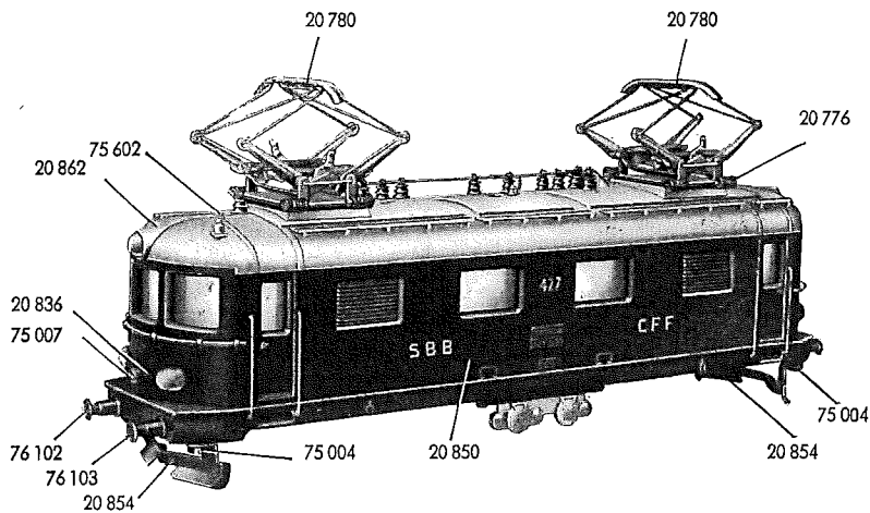
Fig. 1 Lokomotiv-Aufbau
