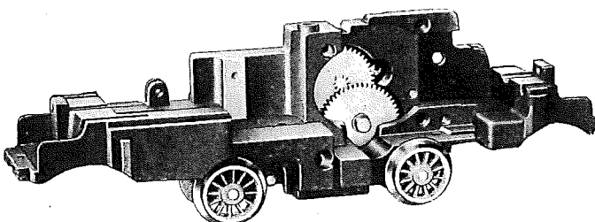
Fig. 3 Treibgestell
