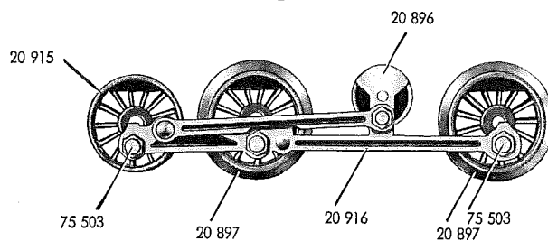
Fig. 7 Treibräder mit Gestänge
