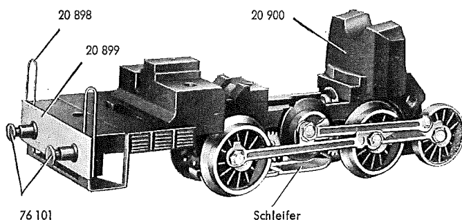
Fig. 4 Treibgestell
