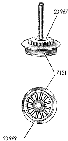
Fig. 5 Treibachsenteil und Treibrad
