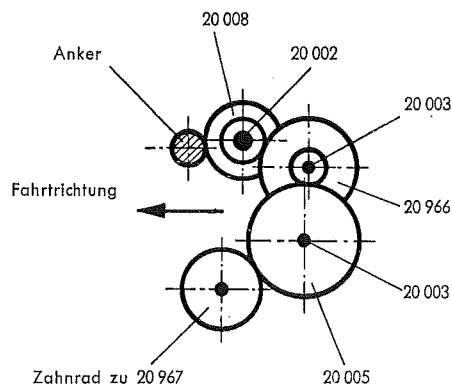
Fig. 4 Anordnung der Getrieberäder
