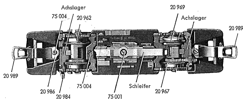
Fig. 2a Fahrgestell von unten gesehen
