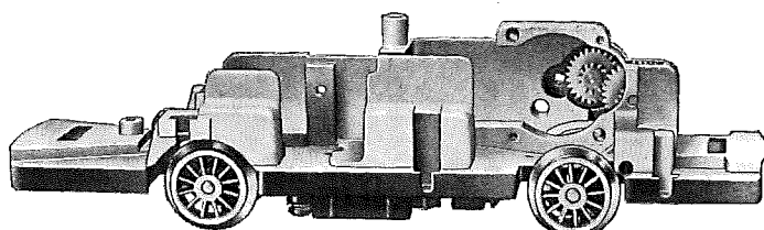
Fig. 3 Treibgestell
