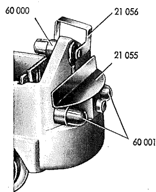
Fig. 2a Endbeleuchtung
