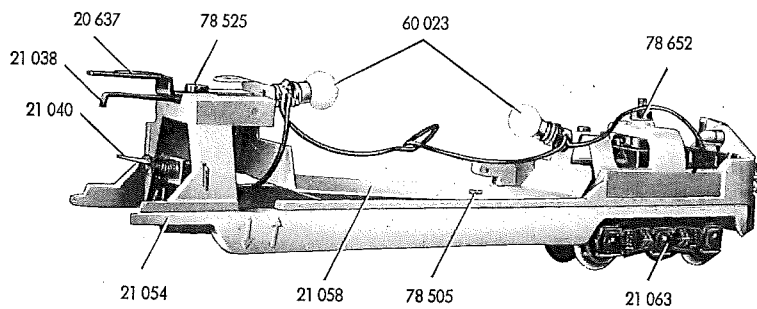
Fig. 2 Hinteres Fahrgestell
