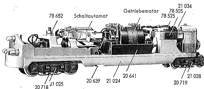
Fig. 2 Vorderwagen
