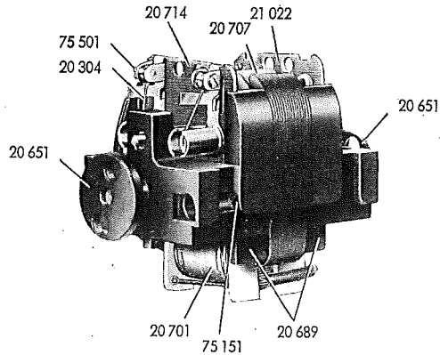
Fig. 3 Getriebemotor
