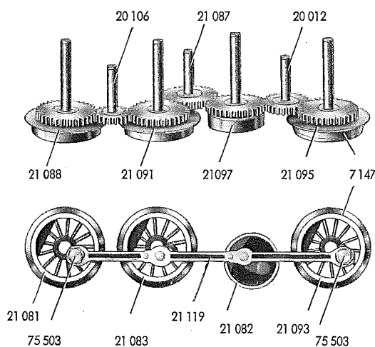
Fig. 6 Laufgestell
