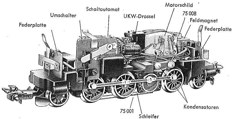
Fig. 2 Fahrgestell
