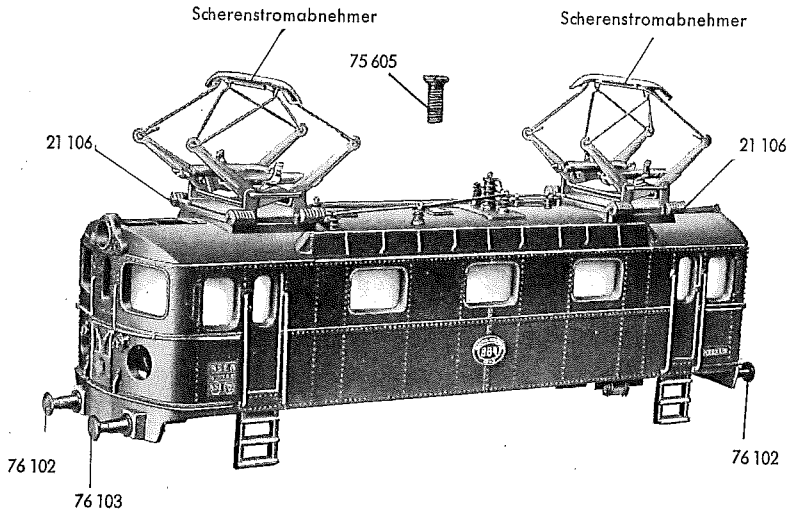
Fig. 1 Lokomotiv-Aufbau
