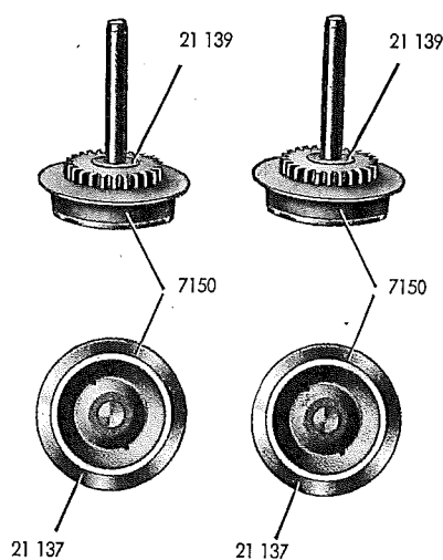
Fig. 5 Treibachse mit Treibrad
