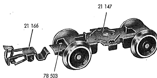
Fig. 7 Stromzuführung
