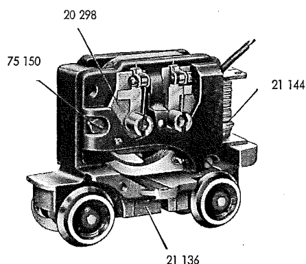
Fig. 3 Getriebemotor (ohne Entstöratz)
