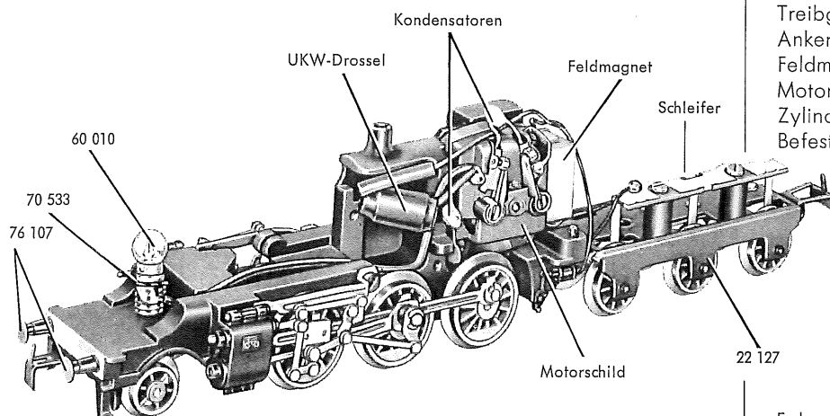
Fig. 2 Fahrgestell mit Tenderfahrgestell
