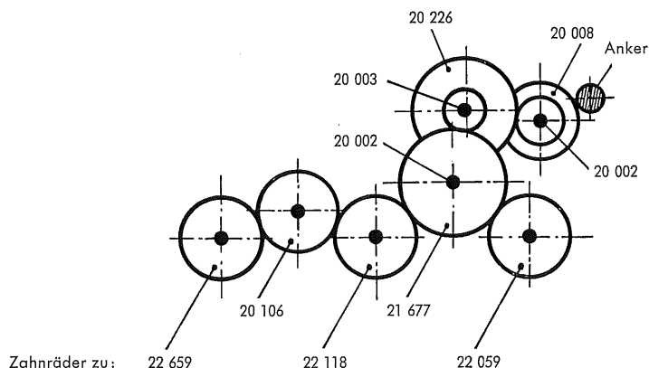
Fig. 5 Treibachse und Treibräder
