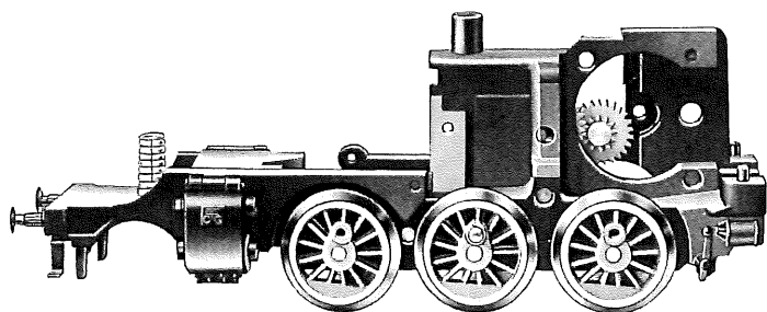
Fig. 3 Treibgestell
