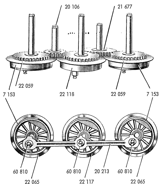
Fig. 5 Treibachse und Treibräder
