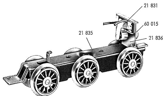
Fig. 7 Drehgestell
