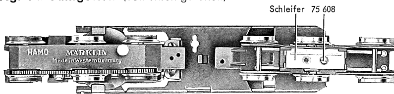
Fig. 4 Motordrehgestell
