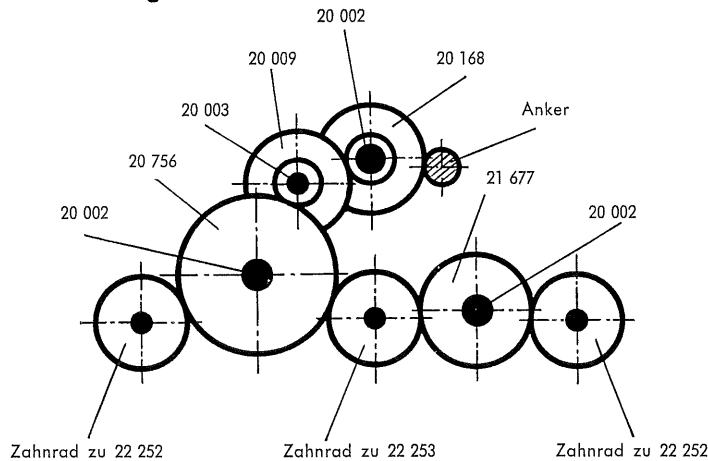
Fig. 6 Treibachsteile und Treibräder
