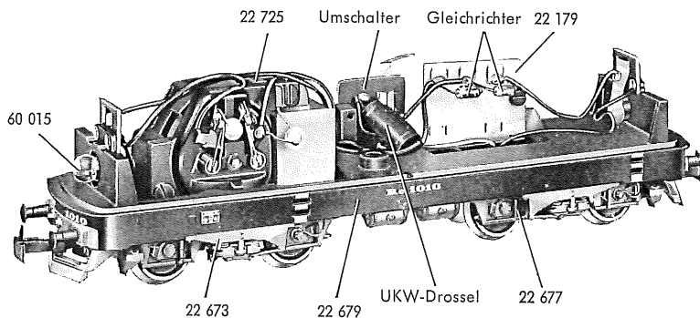
Fig. 2 a Fahrgestell (von unten gesehen)
