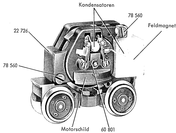
Fig. 3 Motordrehgestell
