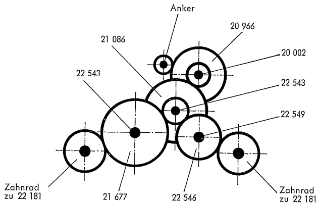
Fig. 4 Anordnung der Getrieberäder
