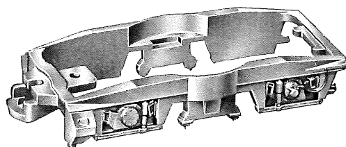
Fig. 7 Drehgestellrahmen (Treibgestell)
