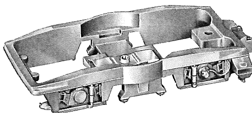
Fig. 10 Drehgestellrahmen (Drehgestell)
