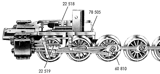
Fig. 6 Gestänge
