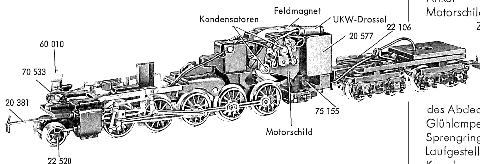
Fig. 2a Fahrgestell mit Tenderfahrgestell (von unten gesehen)
