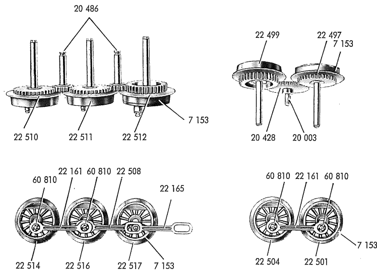
Fig. 5 Treibachsenteile, Treibräder und Kuppelstangenteile
