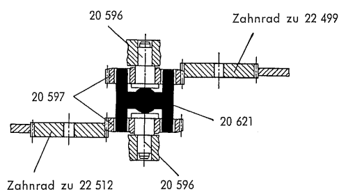
Fig. 4a Getriebekupplung
