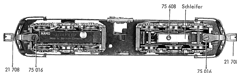
Fig. 3 Motordrehgestell
