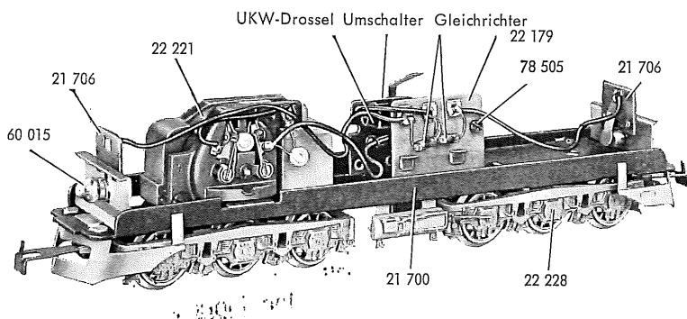
Fig. 2 Fahrgestell
