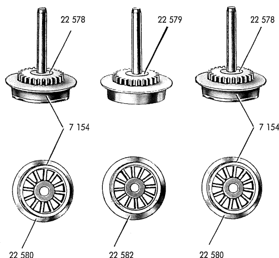
Fig. 5 Treibachsteile und Treibräder
