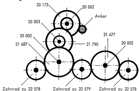
Fig. 5 Treibachsteile und Treibräder
