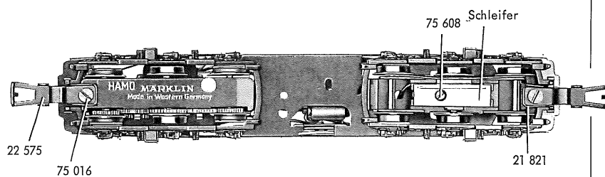
Fig. 3 Motordrehgestell
