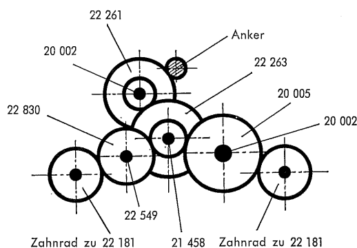
Fig. 5 Treibachsenteil und Treibräder
