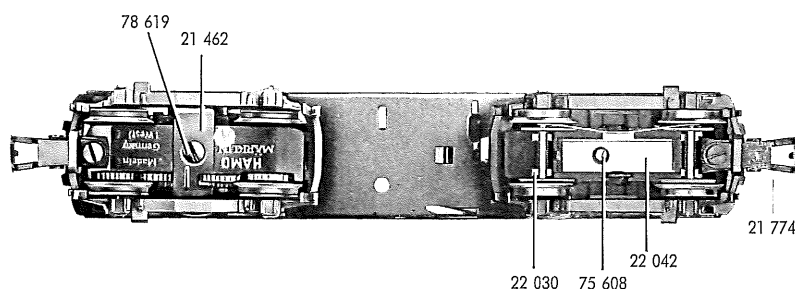
Fig. 2a Fahrgestell (von unten gesehen)
