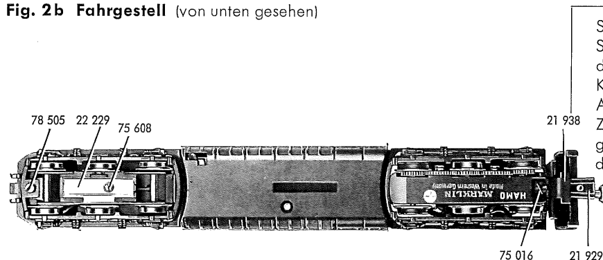
Fig. 2b Fahrgestell (von unten gesehen)
