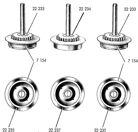
Fig. 5 Treibachsenteil und Treibrad
