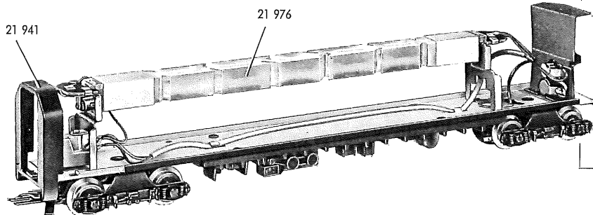
Fig. 13 Fahrgestell
