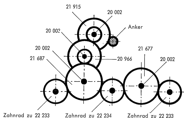
Fig. 5 Treibachsenteil und Treibrad
