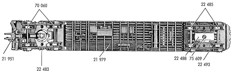
Fig. 14 Kontaktplatte
