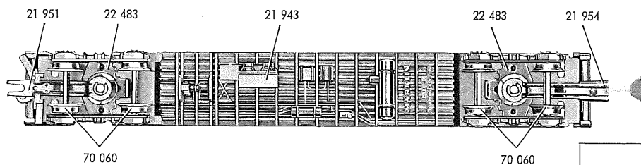
Fig. 11 a Fahrgestell (von unten gesehen)
