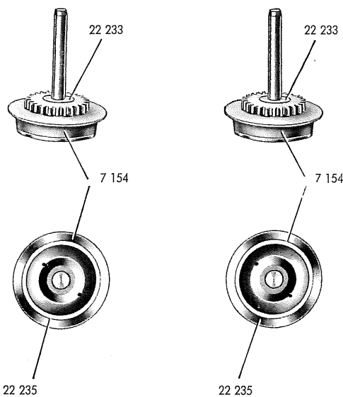
Fig. 5 Treibachsteil und Treibrad
