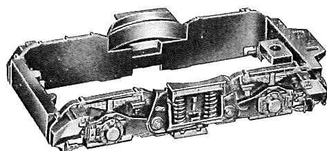
Fig. 8 Drehgestellrahmen (Treibgestell)
