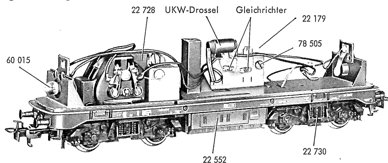
Fig. 2 Fahrgestell
