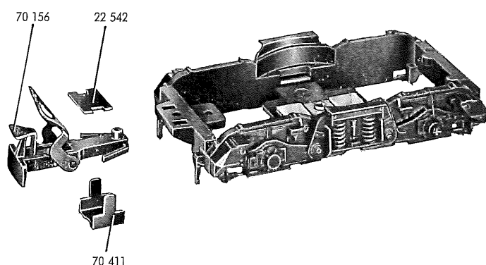
Fig. 7 Drehgestellrahmen (Drehgestell) Kupplung
