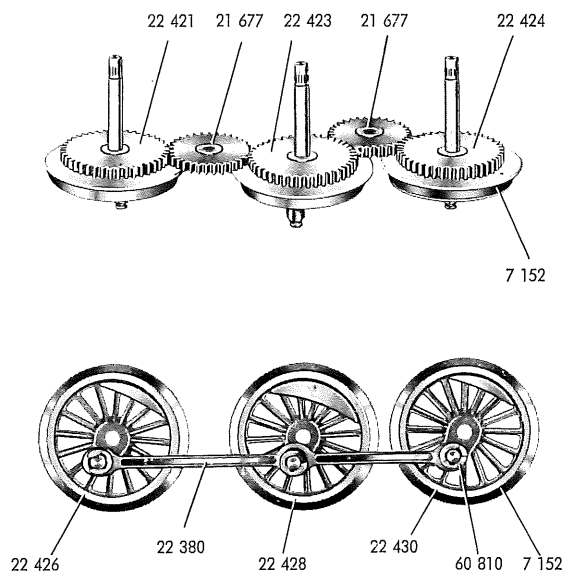
Fig. 5 Treibachsenteile und Treibräder
