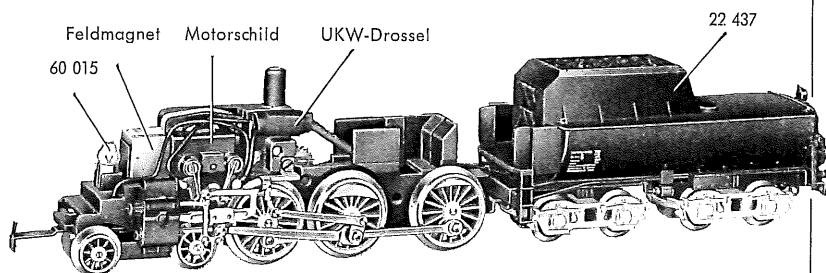
Fig. 2 Fahrgestell mit Tender
