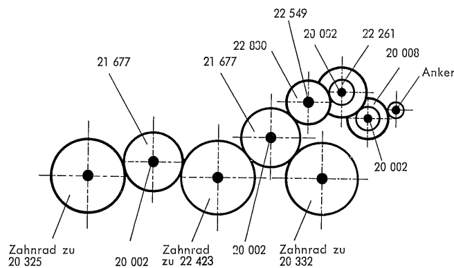
Fig. 5 Treibachsenteile und Treibräder
