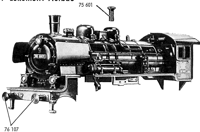
Fig. 1 Lokomotiv-Aufbau
