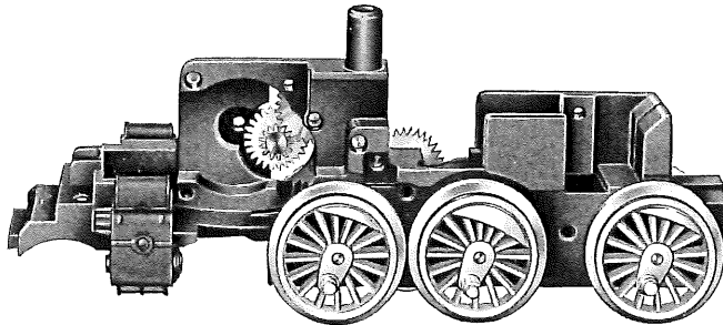
Fig. 3 Treibgestell
