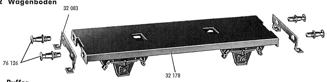
Fig. 2 Wagenboden
