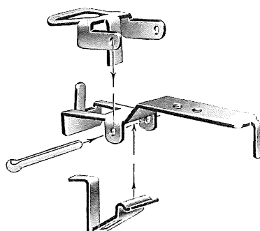
Fig. 7 Zugfeder zur Verbindung der Kupplungen
