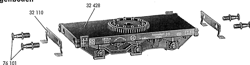
Fig. 4 Wagenboden
