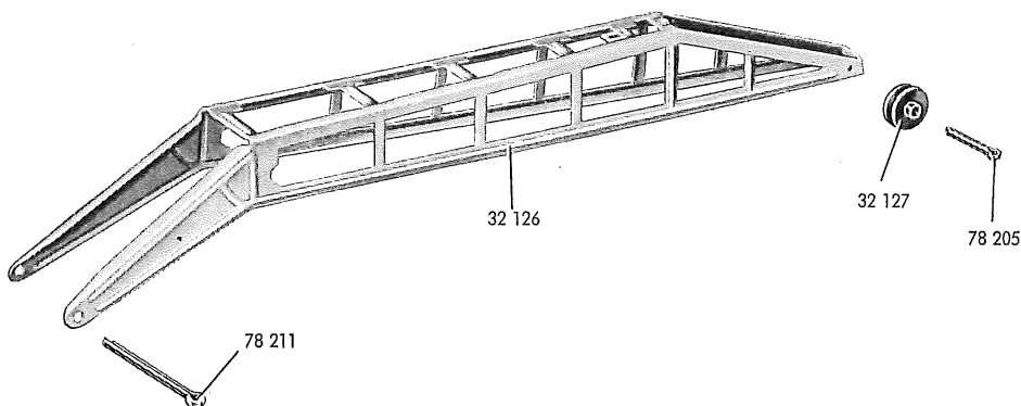
Fig. 5 Ausleger
