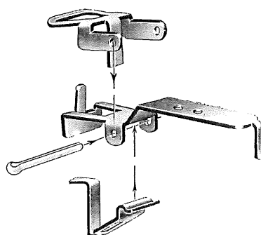
Fig. 10 Kupplung
