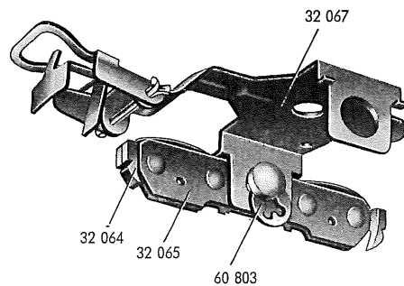
Fig. 3 Drehgestell mit Kupplung (Teilansicht)
