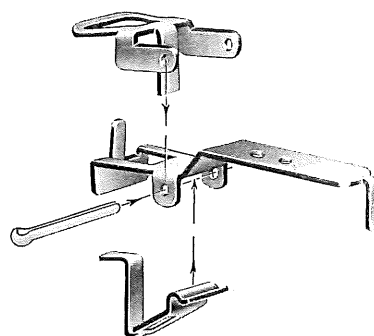
Fig. 7 Zugfeder zur Kupplung
