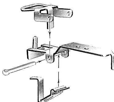
Fig. 10 Zugfeder zur Verbindung der Kupplungen
