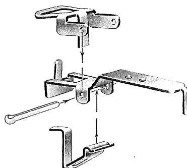
Fig. 9 Zugfeder zur Verbindung der Kupplungen
