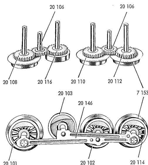
Fig. 5 Treibachsenteile und Treibräder
