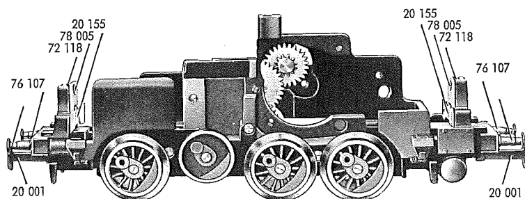
Fig. 3 Treibgestell
