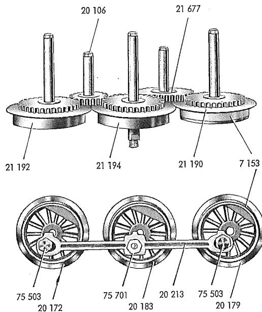
Fig. 5 Treibachsenteile und Treibräder
