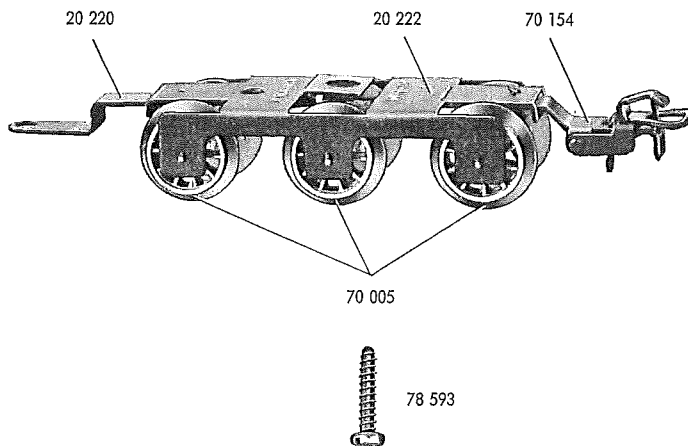
Fig. 2 Fahrgestell
