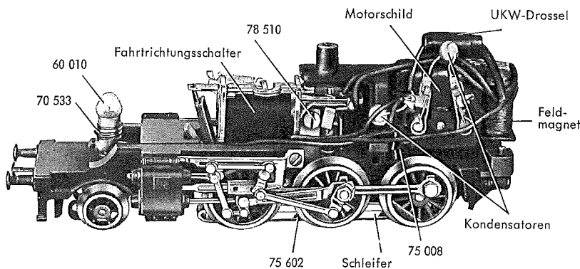
Fig. 3 Treibgestell
