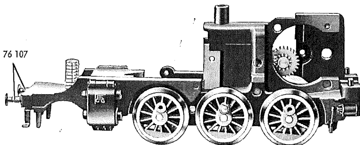
Fig. 3 Treibgestell
