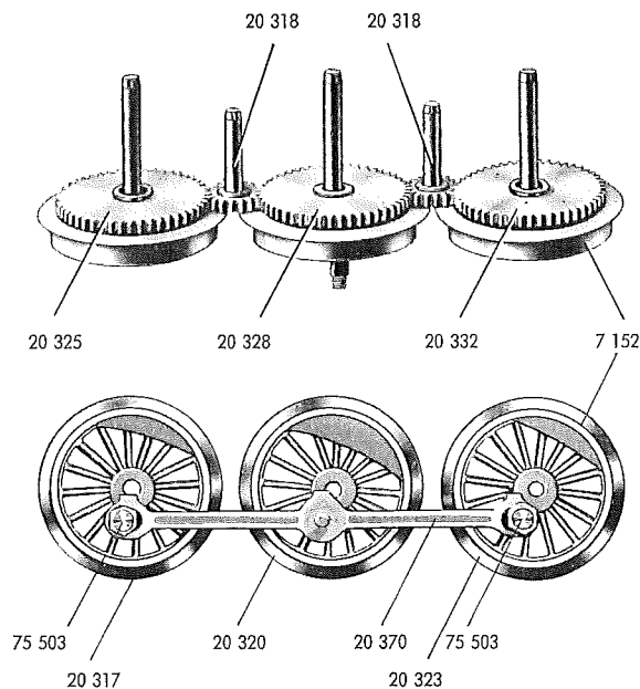
Fig. 5 Treibachsenteile und Treibräder
