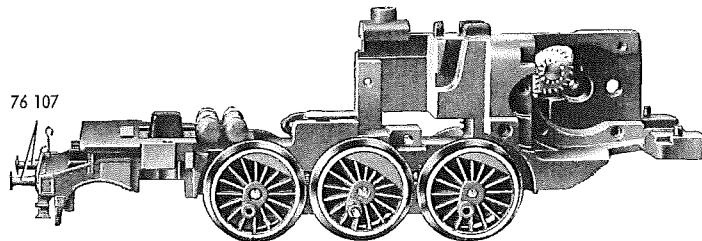
Fig. 4 Anordnung der Getrieberäder
