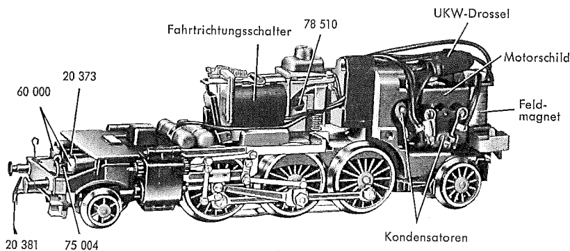
Fig. 2 Fahrgestell
