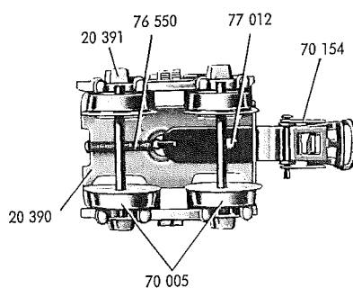
Fig. 3 Drehgestell mit Kupplung (von unten gesehen)
