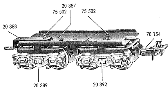
Fig. 2 Fahrgestell
