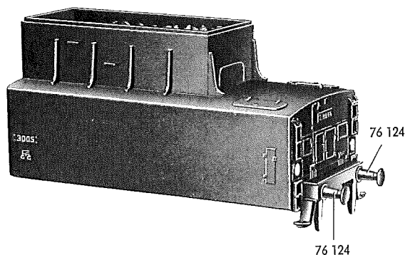
Fig. 1 Tender-Aufbau
