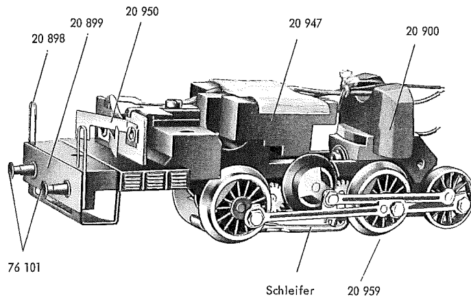
Fig. 4 Treibgestell (Beschwerung)
