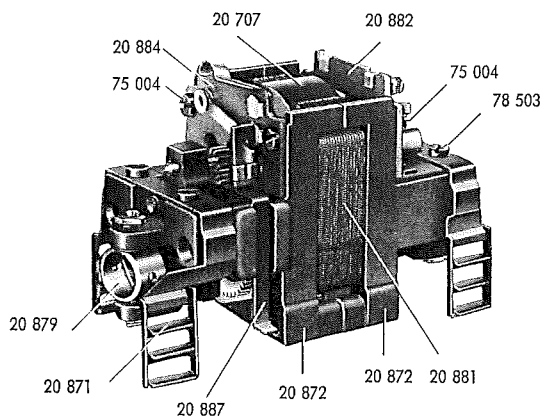
Fig. 3 Getriebemotor
