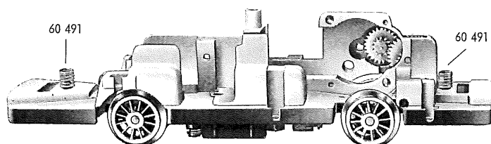
Fig. 3 Treibgestell
