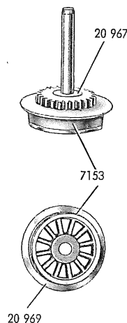
Fig. 7 Kupplung
