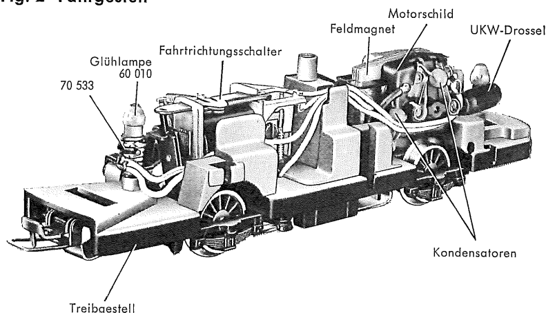
Fig. 2 Fahrgestell
