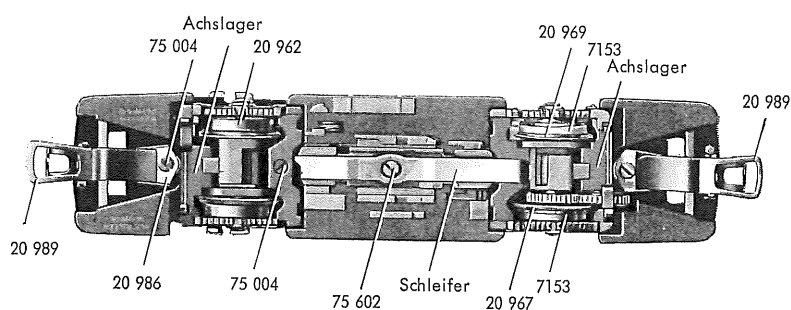
Fig. 2a Fahrgestell (von unten gesehen)
