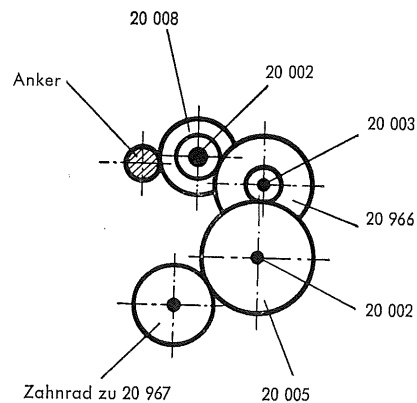
Fig. 5 Treibachsenteil und Treibrad
