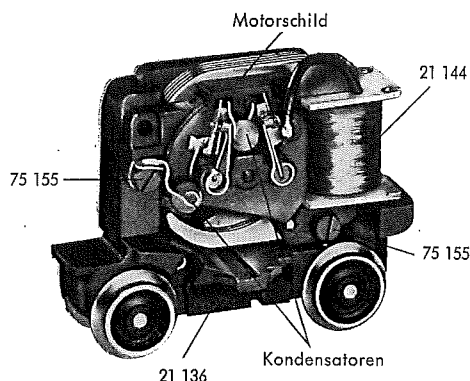
Fig. 3 Getriebemotor
