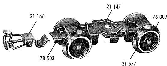
Fig. 7 Drehgestellrahmen (zum Getriebemotor)
