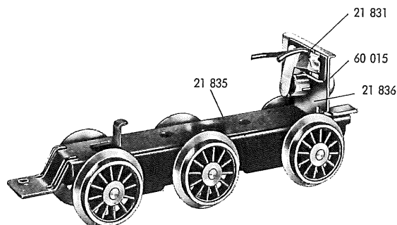
Fig. 7 Drehgestell
