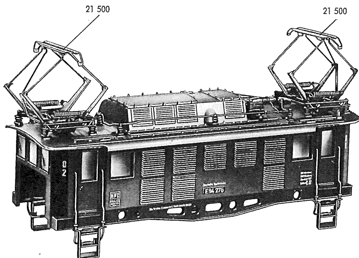
Fig. 1 Lokomotiv-Aufbau
