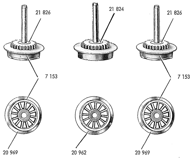
Fig. 6 Treibachsteile und Treibräder
