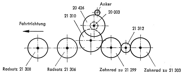
Fig. 4 Anordnung der Getrieberäder
