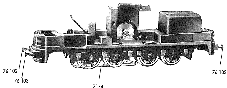
Fig. 3 Treibgestell
