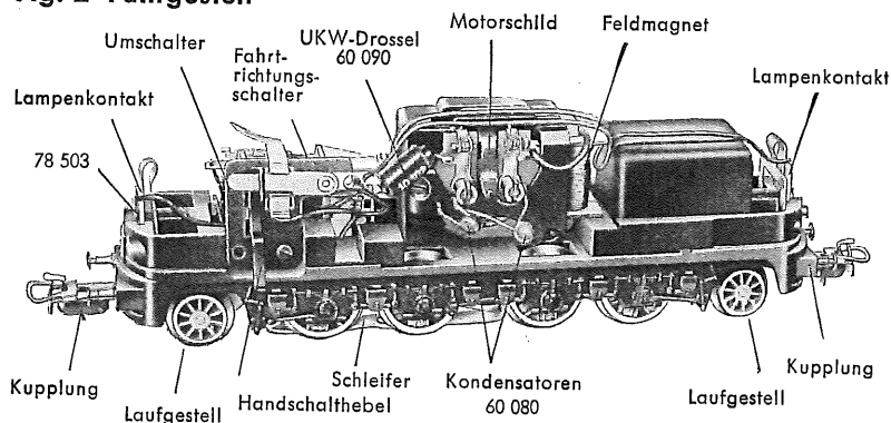
Fig. 2 Fahrgestell
