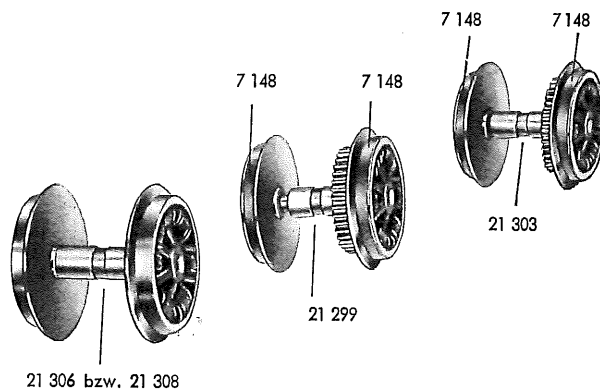
Fig. 5 Treibradsätze und Radsätze
