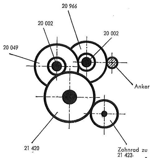
Fig. 4 Anordnung der Getrieberäder
