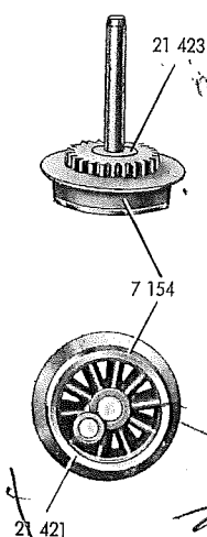
Fig. 5 Treibachsenteil und Treibrad
