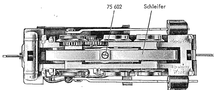
Fig. 3 Treibgestell
