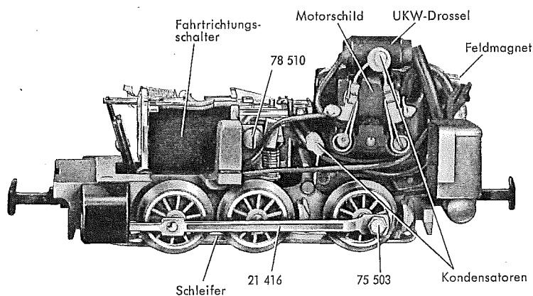
Fig. 2 Fahrgestell
