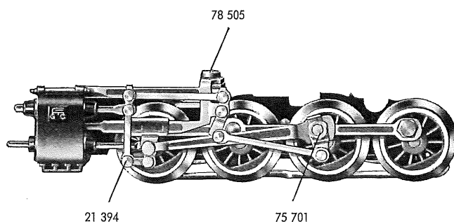
Fig. 6 Gestänge
