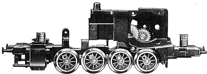
Fig. 3 Treibgestell
