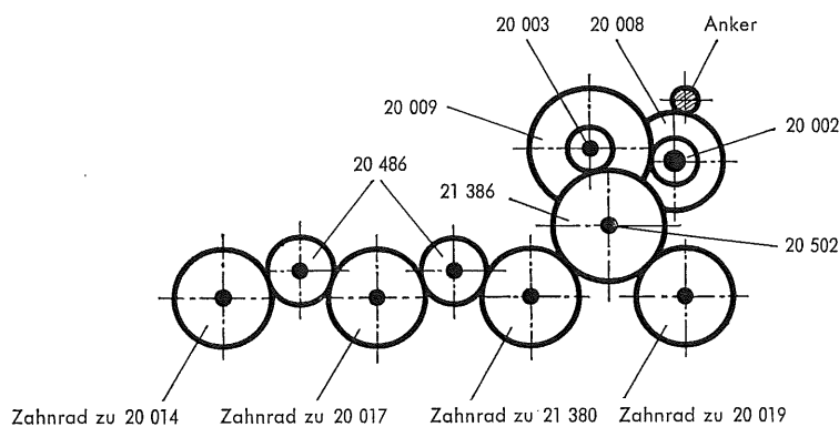
Fig. 5 Treibachsenteile und Treibräder
