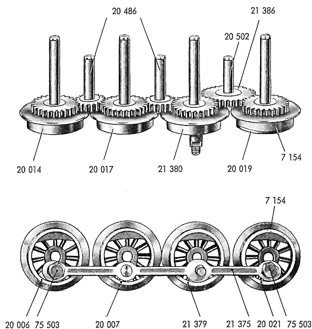
Fig. 5 Treibachsenteile und Treibräder
