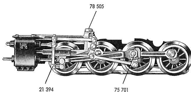
Fig. 6 Gestänge
