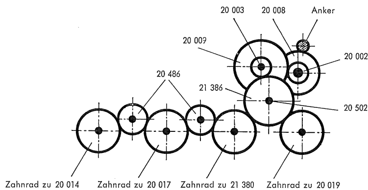
Fig. 5 Treibachsenteile und Treibräder
